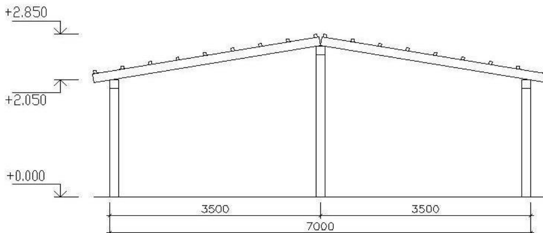
Рисунок 2 Разрез с высотными отметками
